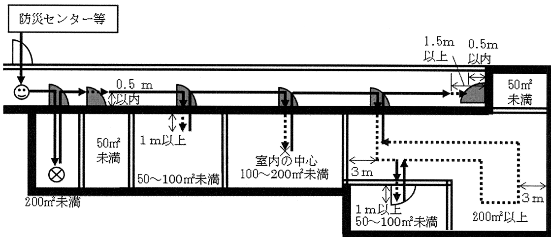
図1 防火区画外の通路から確認する方法（例）
